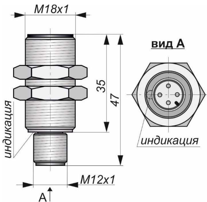
Габаритный чертеж
